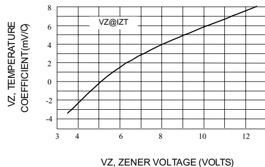
Fig. 2-ZENER VOLTAGE- 5.1 TO 12 VOLTS
