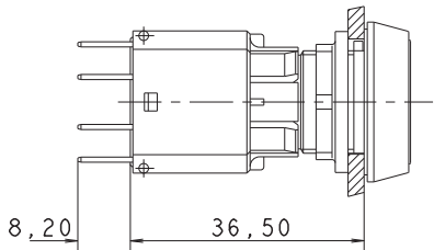
Leuchtvorsatz mit Lampenfassung
