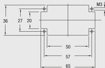
Montageausschnitt/ Panel cut-out
