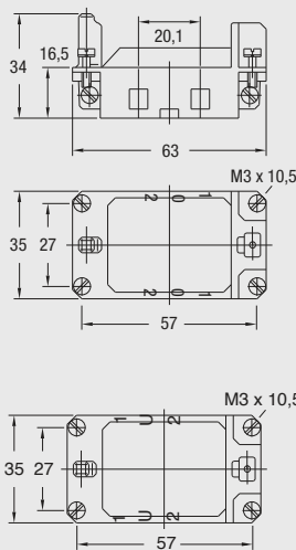
Montageausschnitt/ Panel cut-out
