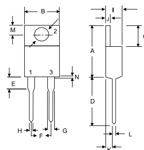
TO-220A
