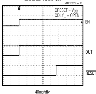
ENABLE TURN-ON
