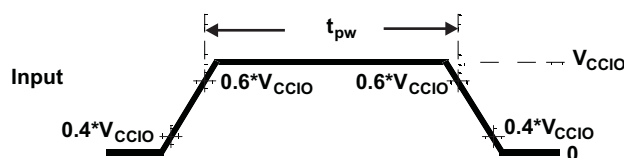
Figure 5-8. FlexRay Inputs
