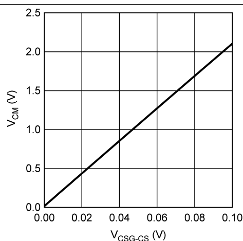
Figure 14. V_{CM} vs V_{CSG-CS}
