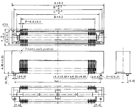
Unit:mm
