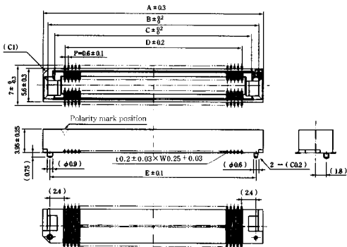
Unit:mm
