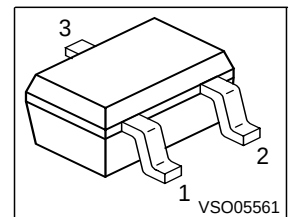
PG-SOT-323
