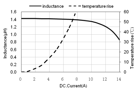
ASPIAIG-S8050-1R5
