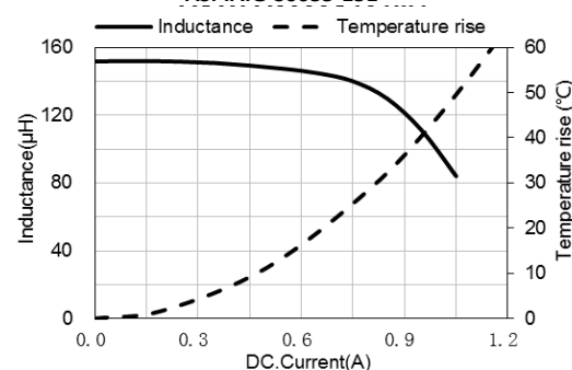
ASPIAIG-S6055-151
