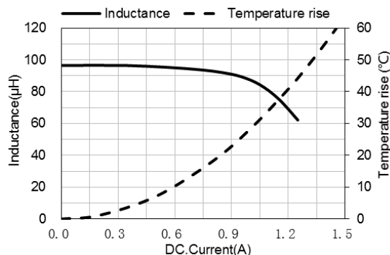
ASPIAIG-S6055-101
