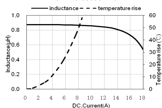
ASPIAIG-S8050-1R0
