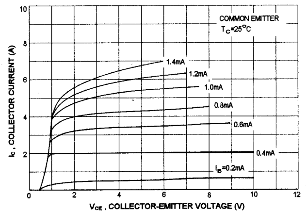
I_C - V_{CE}
