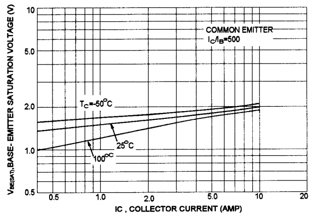
V_{BE(sat)} - I_C
