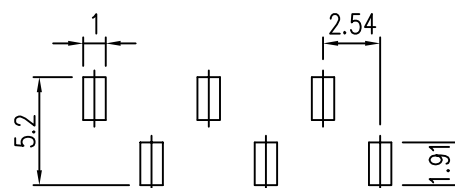
P.C.B LAYOUT
