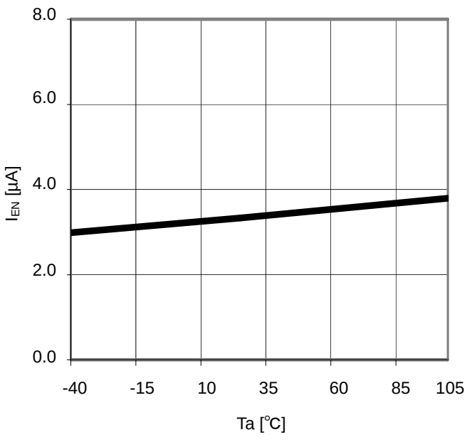
Figure 24. Ta-I EN
