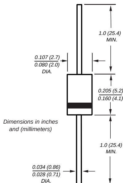
DO-204AL (DO-41)
