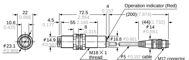
CY-19□-J Sensor
