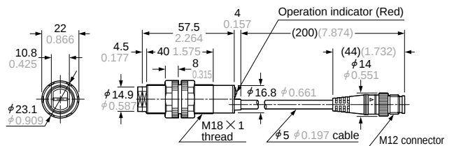
CY-29□-J Sensor
