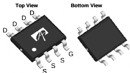
SOIC-8
