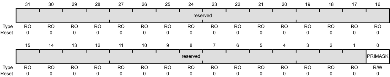
Priority Mask Register (PRIMASK)
