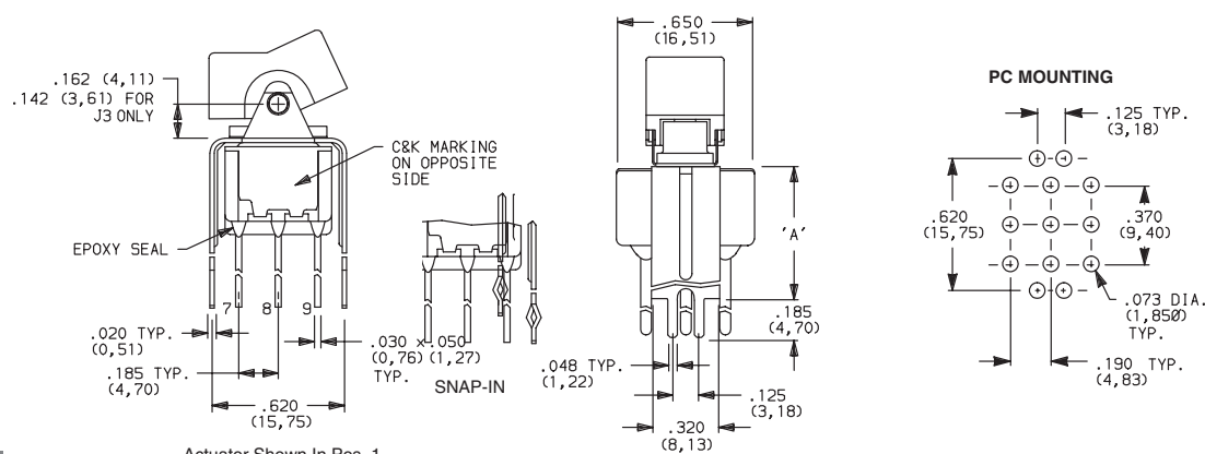
7301J1_BE2 3PDT
