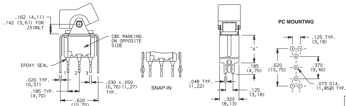
7101J1_BE2 SPDT
