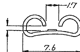
断面 A~A
