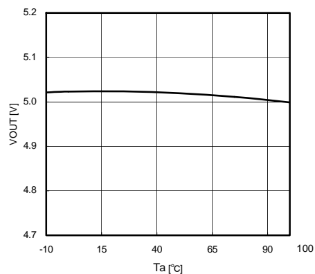
Fig.7 T_a - V_o ( I_o=0\text{mA} )
