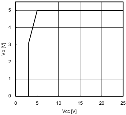
Fig.13 Vcc-Vo
