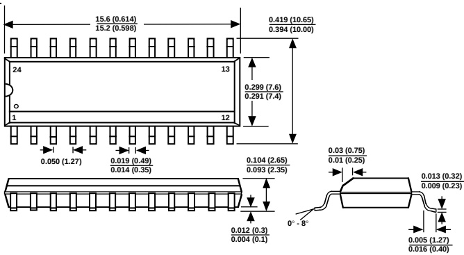
SOIC (R-24)
