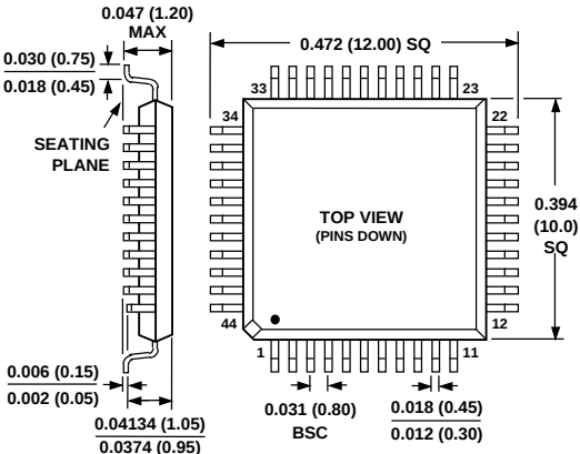
TQFP (ST-44B)
