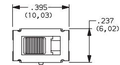
ACTUATOR IN POS. 1
