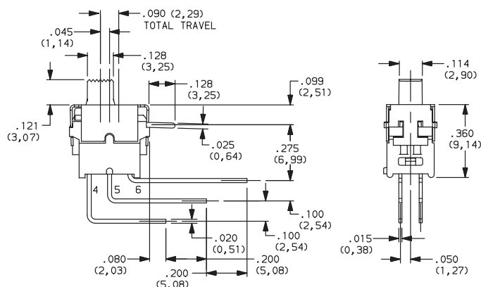
ES21MAVKE DPDT
