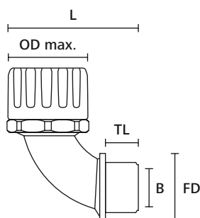
HelaGuard koppling, 90° med fast utvändig gänga
