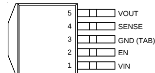
TO-263-5 RT9172S-□□xM5
