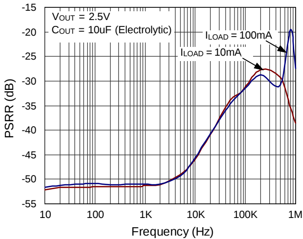
PSRR
