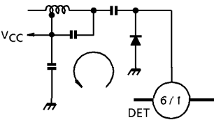
Fig.4 Rectifier loop
