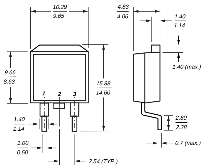
TO-263
