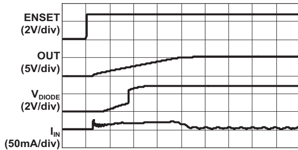
Turn-On
