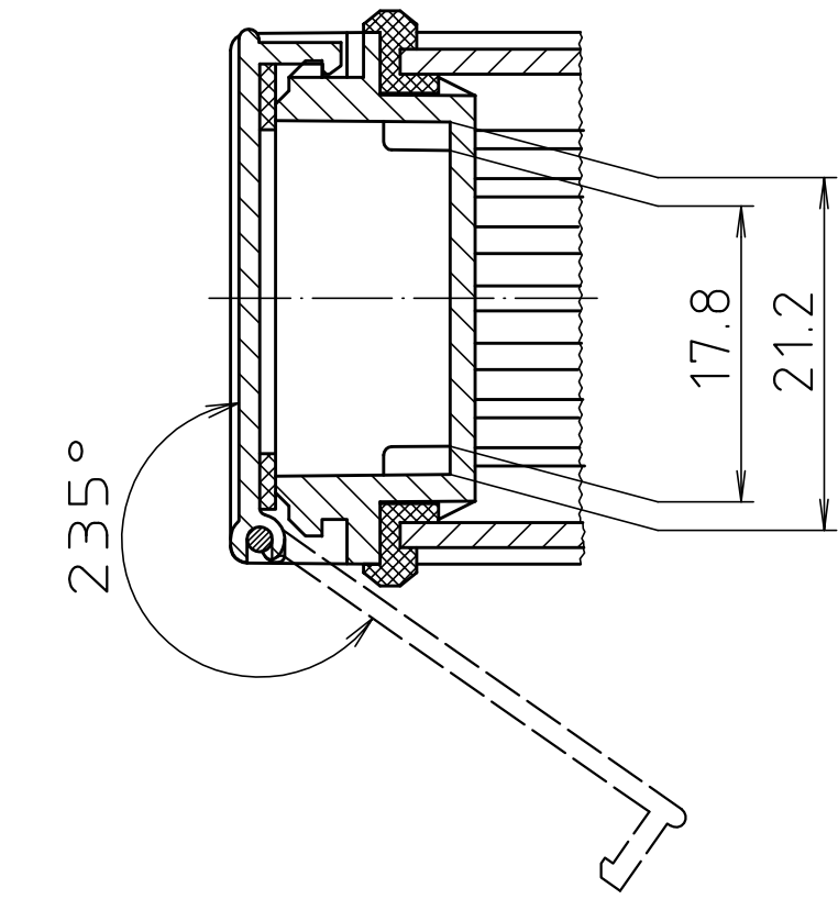
ABM 800 ... BE (weitere Masse siehe ABM 800 ... / more dimensions see ABM 800 ...)
