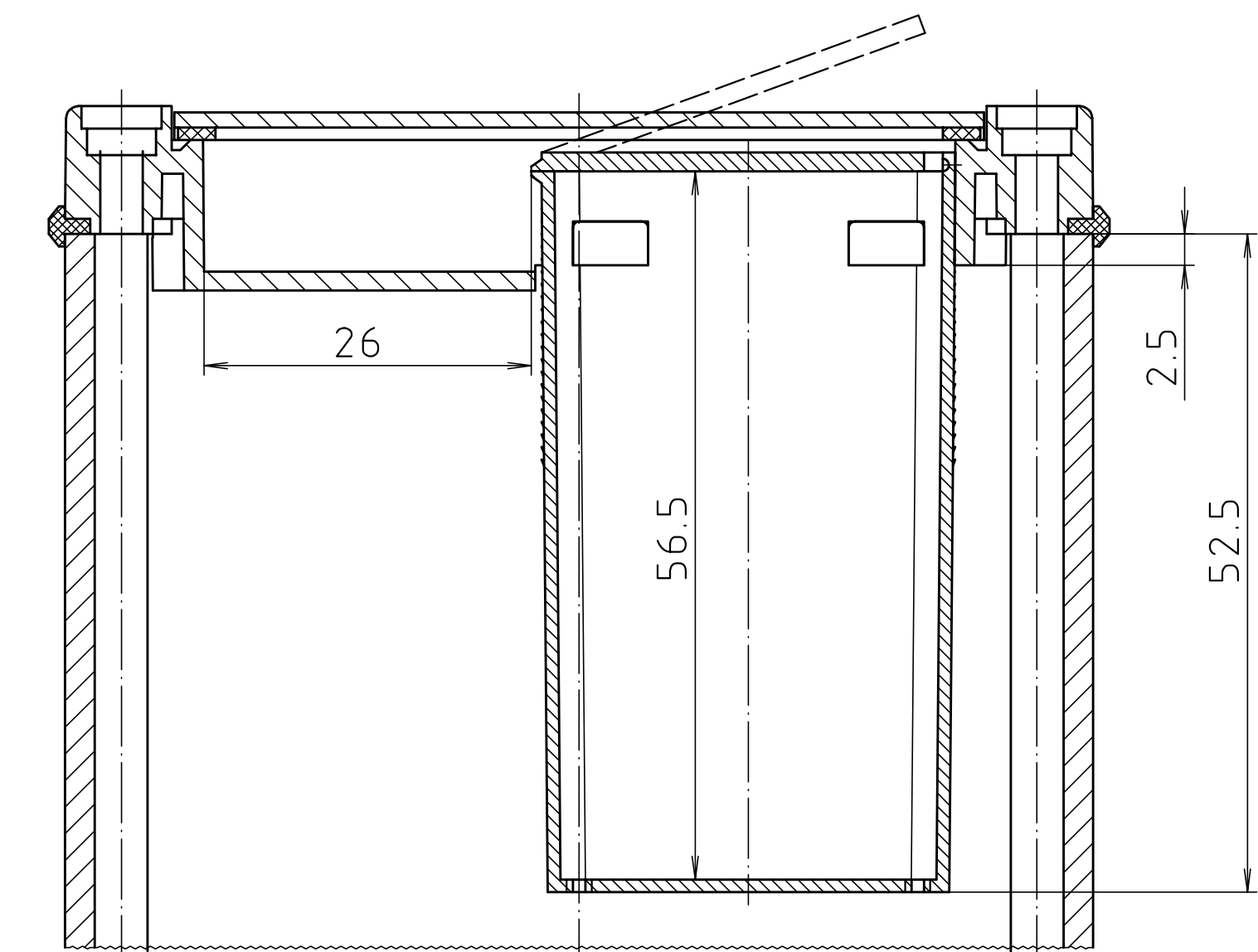
ABM 800 ... BE (weitere Masse siehe ABM 800 ... / more dimensions see ABM 800 ...)
