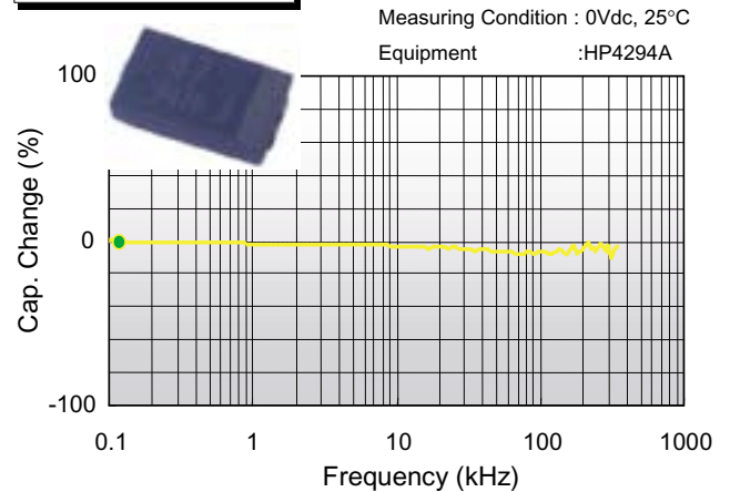
TA (Y) 2917/47uF/6.3V
