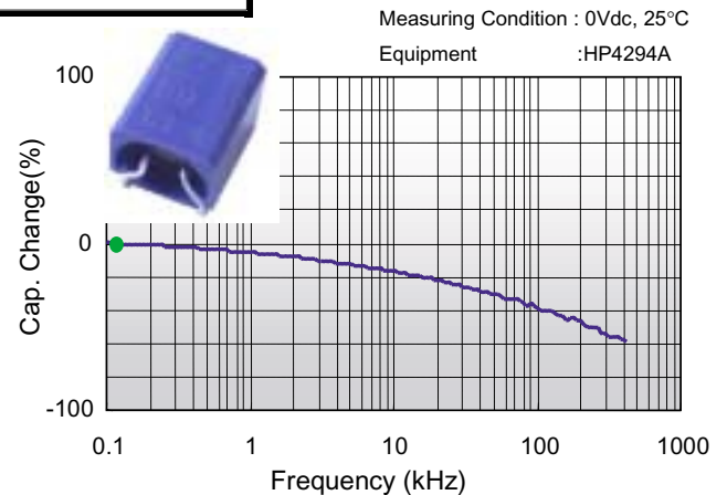
Organic 3628/47uF/10V
