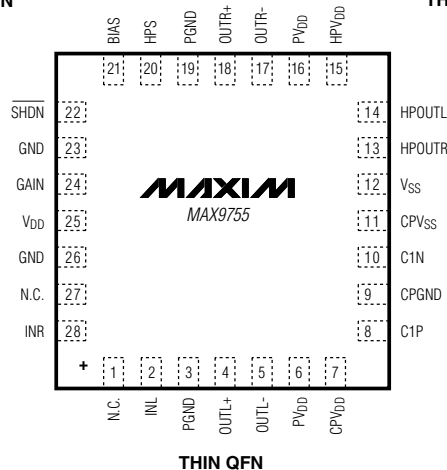
THIN QFN
