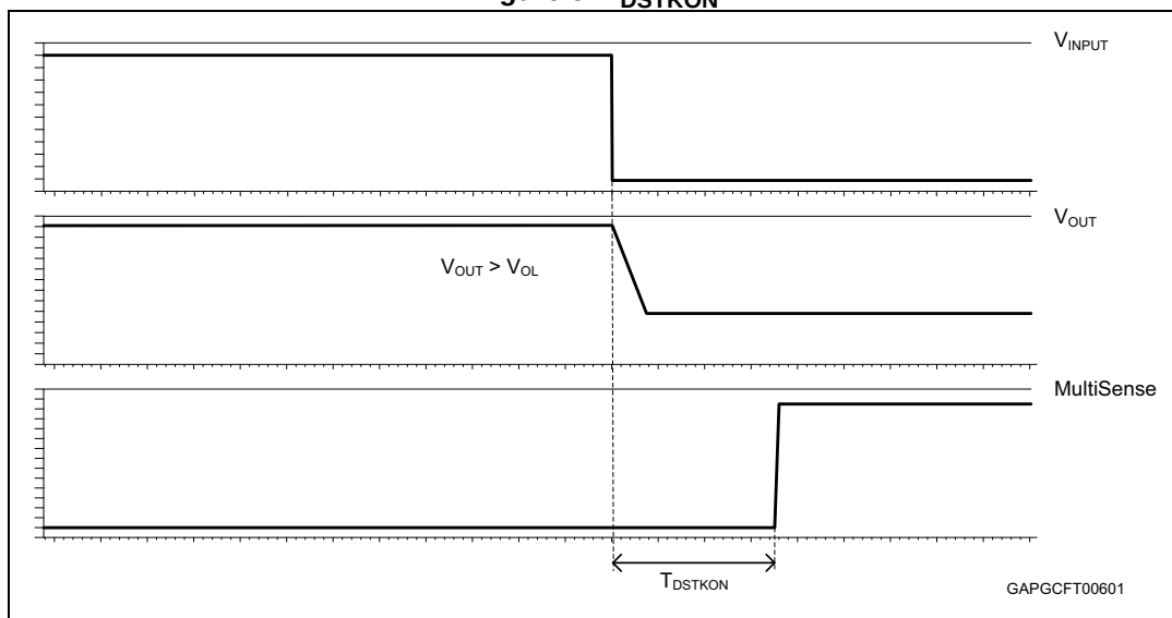
Figure 9. T_{DSTKON}
