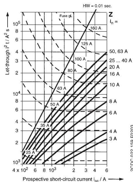
Miniature circuit-breakers S 200 Z
