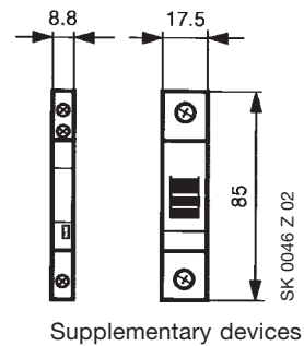
S2C-S/H 6 R S2C-A... S2C-H 6 R S2C-UA...
