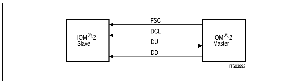
Figure 31 IOM ® -2 Interface Structure
