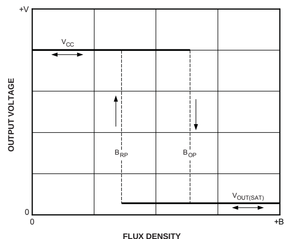
Dwg. GH-007-2
