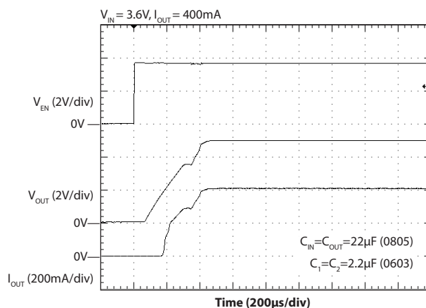
Startup (400mA)
