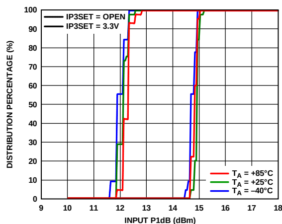
Figure 30. Input P1dB
