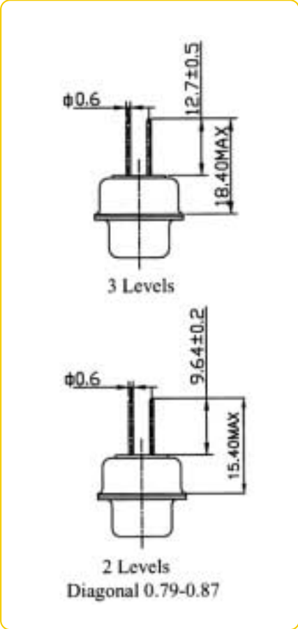
Wire wrap
