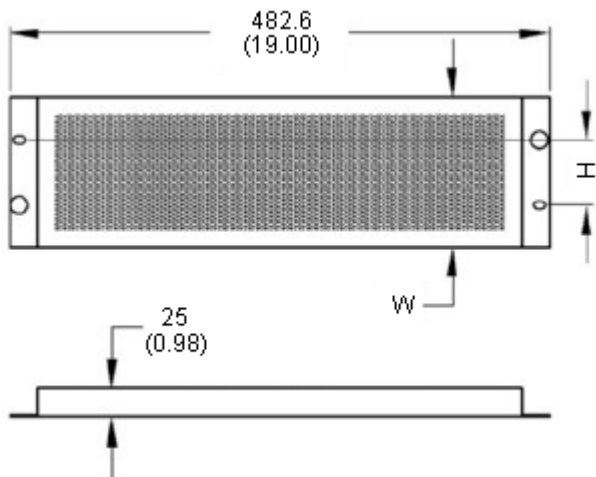
Dimensions : Millimetres (inches)
