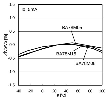
Fig.10 T_a - V_o
