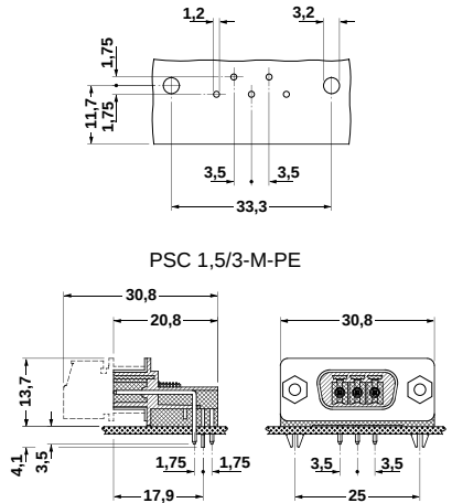
PSC 1,5/3-M-PE
