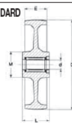
CUSCINETTO A RULLINI STANDARD O INOX - STANDARD OR STAINLESS STEEL ROLLER BEARING - STANDARD ODER ROSTFREIES ROLLENKORBLAGER - ROULEMENT À ROULEAUX STANDARD OU INOX - COJINETE A RODILLOS STANDARD O INOX
