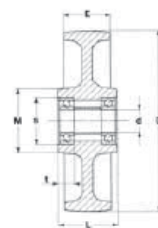
CUSCINETTO A RULLINI STANDARD O INOX - STANDARD OR STAINLESS STEEL ROLLER BEARING - STANDARD ODER ROSTFREIES ROLLENKORBLAGER - ROULEMENT À ROULEAUX STANDARD OU INOX - COJINETE A RODILLOS STANDARD O INOX
