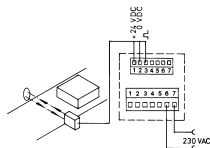
Commande par barrière de lumière
