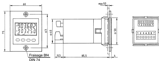
903 avec cadre frontal Nr. 3 Découpe 50 x 50 mm
