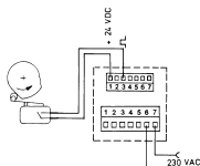
Ansteuerung über Kontakt programmierte Polarität PNP
