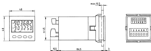
903 Découpe 45 x 45 mm
