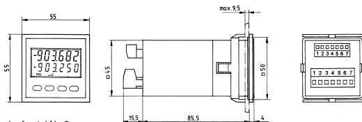
903 avec cadre frontal Nr. 2 Découpe 50 x 50 mm
