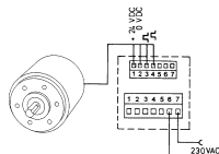
Commande par générateur d'impulsions
