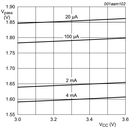
Fig. 5. Pass voltage versus supply voltage; T amb = 125 °C (typical)
