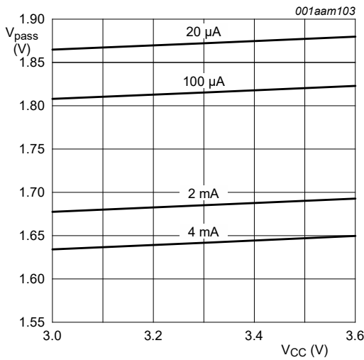
Fig. 6. Pass voltage versus supply voltage; T amb = 85 °C (typical)
