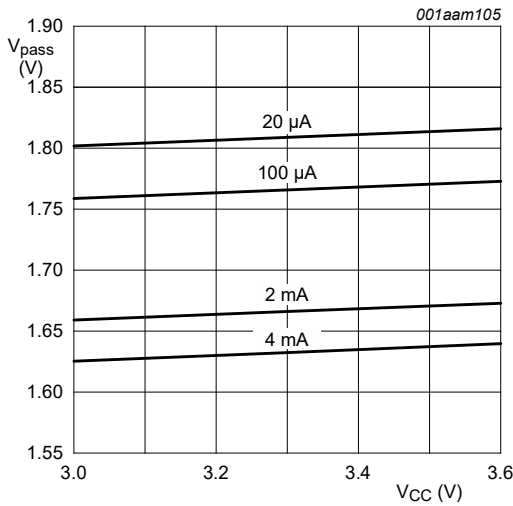
Fig. 8. Pass voltage versus supply voltage; T amb = 0 °C (typical)
