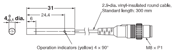
E2E-S04N02-CJ-□□
