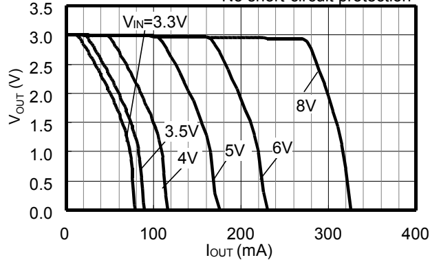
S-812C30A (Ta=25°C)
