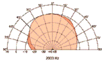
Abstrahlcharakteristik 2000 Hz
