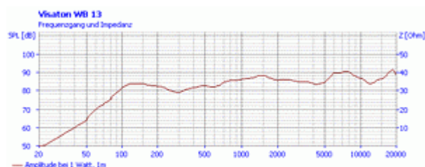
Amplitudenfrequenzgang
