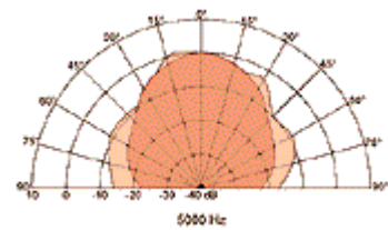
Abstrahlcharakteristik 5000 Hz
