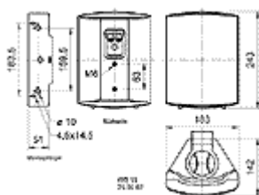
Bauzeichnung
