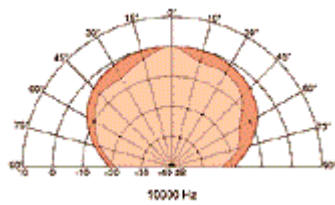
Abstrahlcharakteristik 10000 Hz
