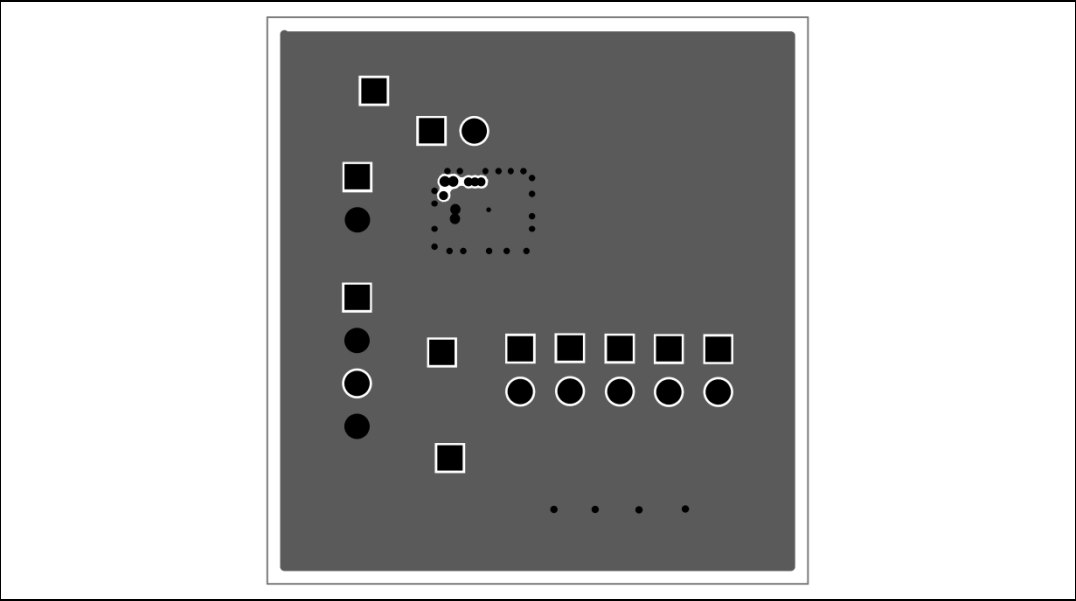
Figure 23. Bottom layer
