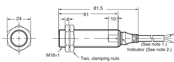
E2AU-M18LS08-WP-□□
