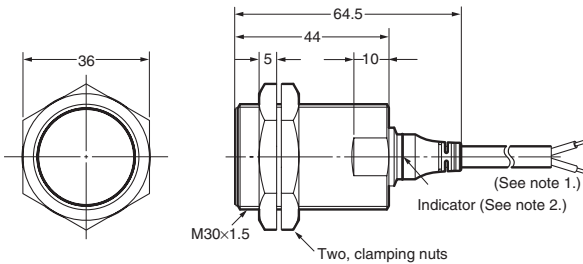
E2AU-M30KS15-WP-□□
