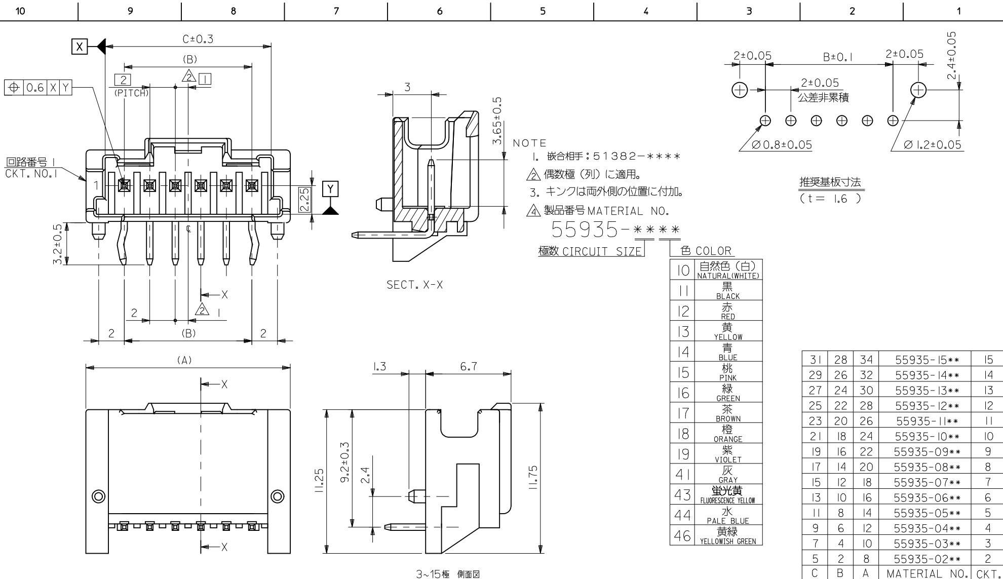
3~15極 側面図
