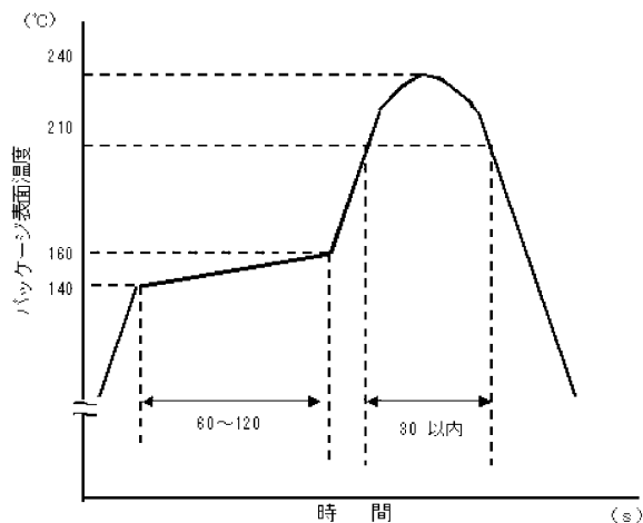
図 13.2.1 共晶はんだ使用時の温度 プロファイル例
