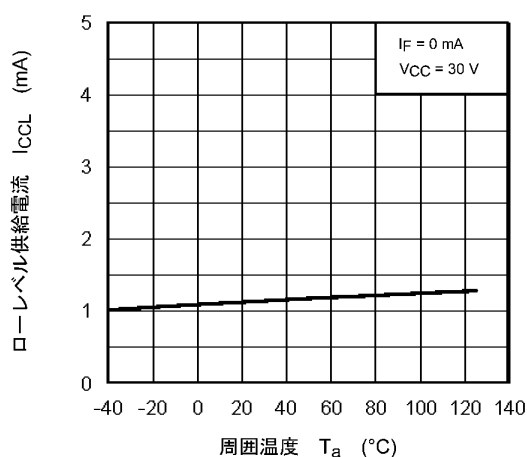
図 12.2.5 I_{CCL} - T_a
