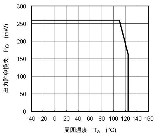
図 12.2.3 P_O - T_a
