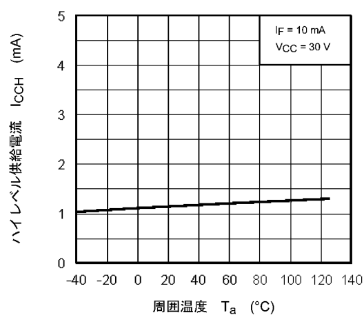
図 12.2.6 I_{CCH} - T_a
