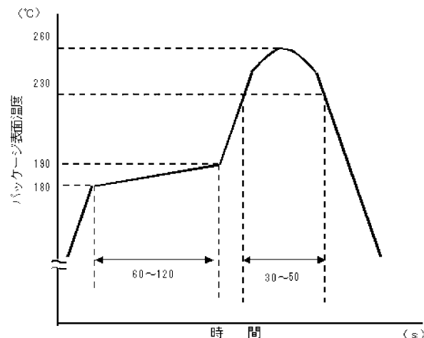
図 13.2.2 鉛フリーはんだ使用時の温度 プロファイル例
