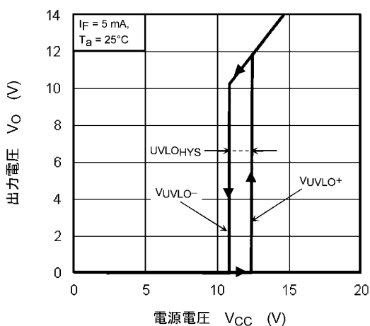
図 12.2.11 V_O(V_{UVLO}) - V_{CC}
