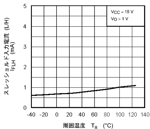
図 12.2.4 I_{FLH} - T_a
