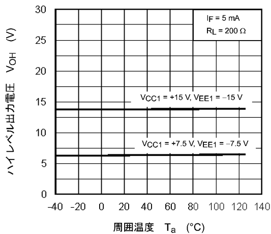
図 12.2.8 V_{OH} - T_a
