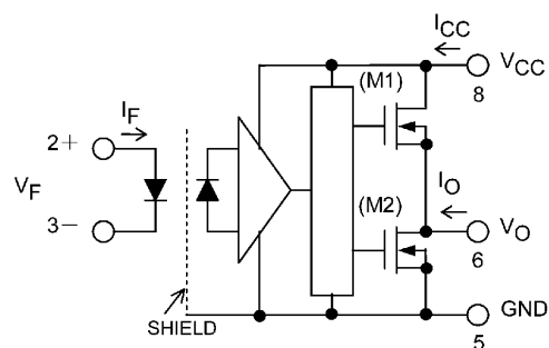
図 5.1 内部回路構成
